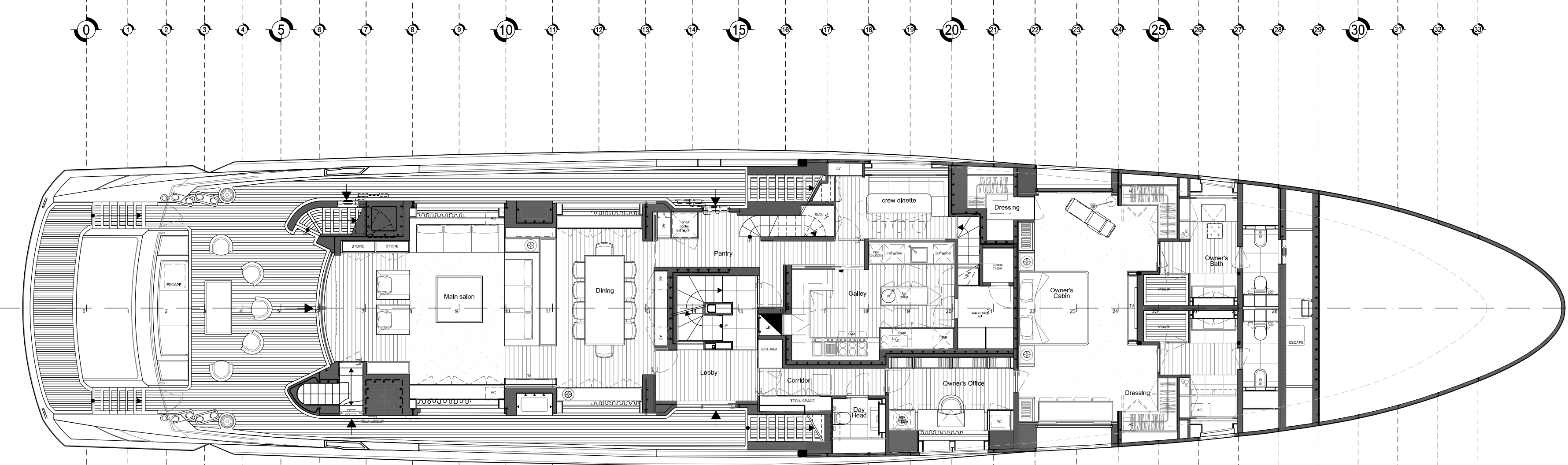
PONTE COPERTA MAIN DECK
