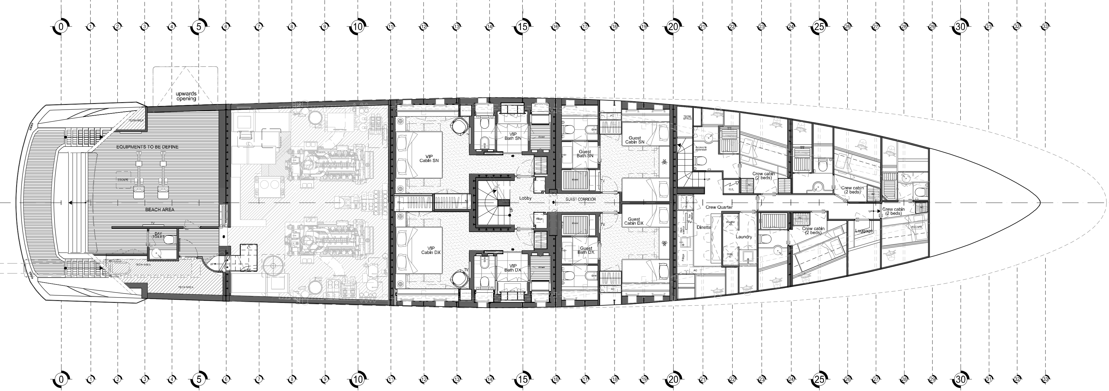
PONTE SOTTOCOPERTA LOWER DECK
